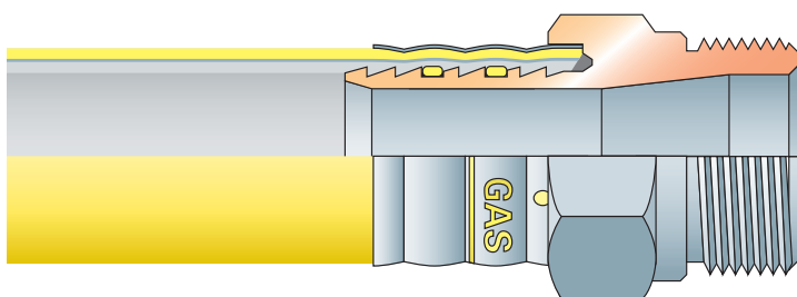
Doorsnedetekening van een Uponor persfitting voor gas, verkrijgbaar in de afmetingen 20, 25 en 32 mm met RVS persschulzen.
